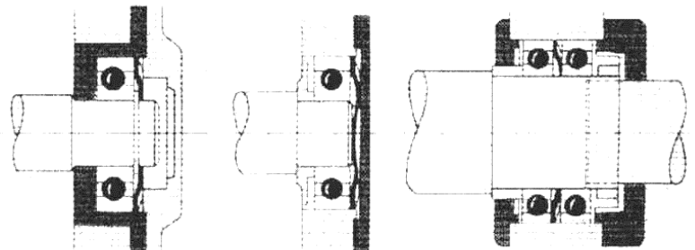
Einbaubeispiele: Kugellagerausgleichsscheiben
